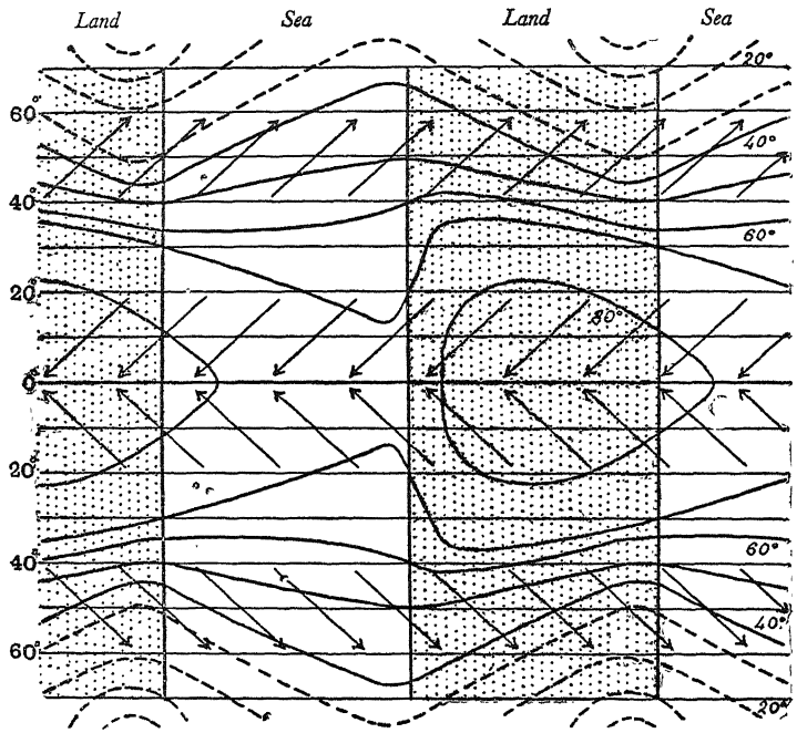
चित्र २८ : समताप रेखाओं के पथ पर हवाओं का प्रभाव
